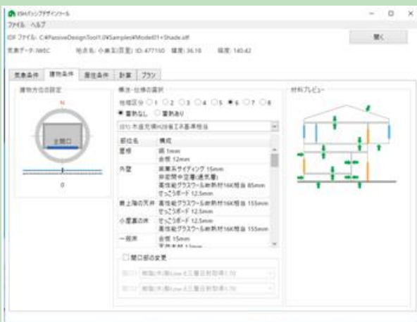
ユーザーインターフェイス／建物条件の設定画面
