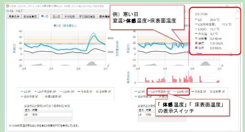
出力結果の例／冬季の室温・体感温度・表面温度(床)
